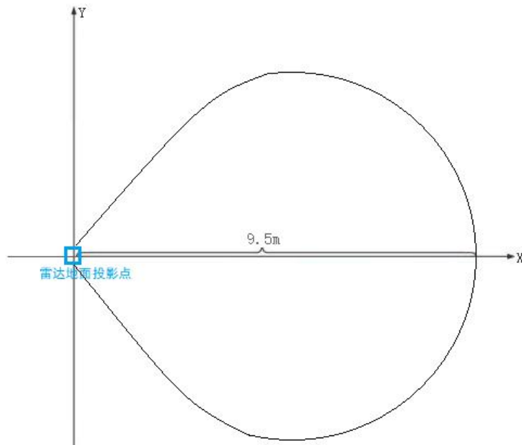
图 2-8 水平安装触发范围
