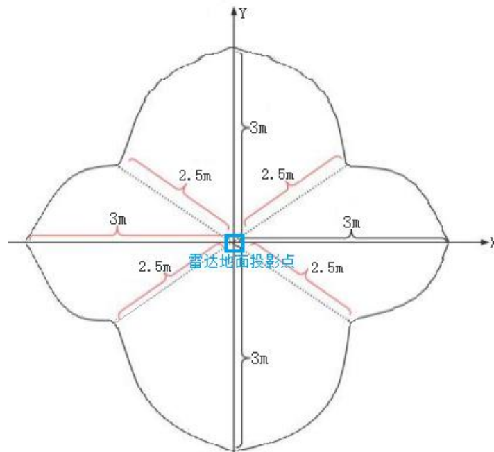
图 2-9 置顶安装极限情况维持范围
