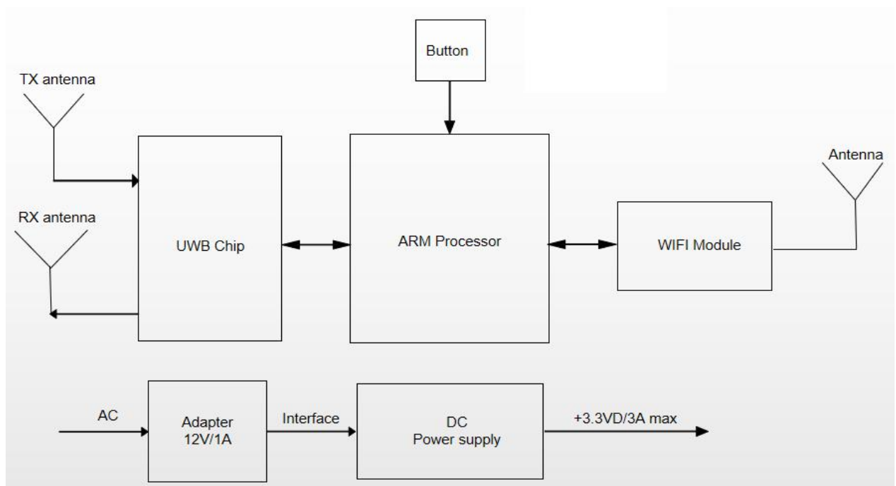
图 1-2 产品方框图
