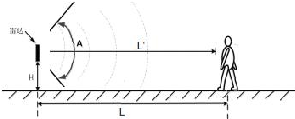
图 2-7 水平安装示意图
