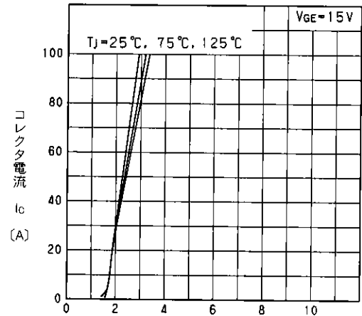
コレクタ・エミッタ間電圧 V_{CE} (V) 飽和電圧-コレクタ電流特性(標準値) V_{CE(sat)} - I_c Characteristics
